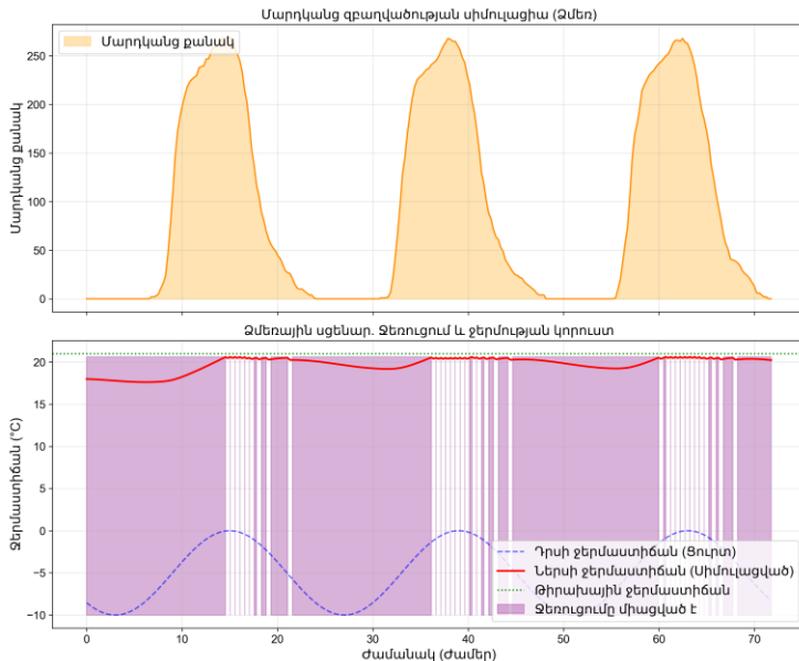
Նկ.1. Ձմեռային շրջանի ջերուցման համակարգի աշխատանքային ռեժիմի սիմուլացիա՝ օգտագործողների զբաղվածության, արտաքին և ներքին ջերմաստիճանների դինամիկա
