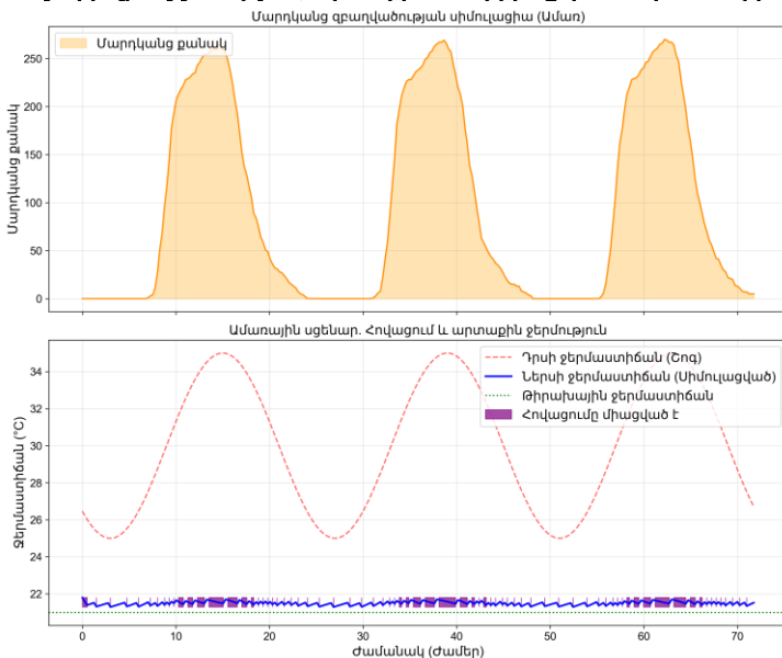
Նկ.2. Ամառային շրջանի կլիմայավորման համակարգի աշխատանքային ռեժիմի սիմուլացիա՝ օգտագործողների զբաղվածության, արտաքին և ներքին ջերմաստիճանների դինամիկա
