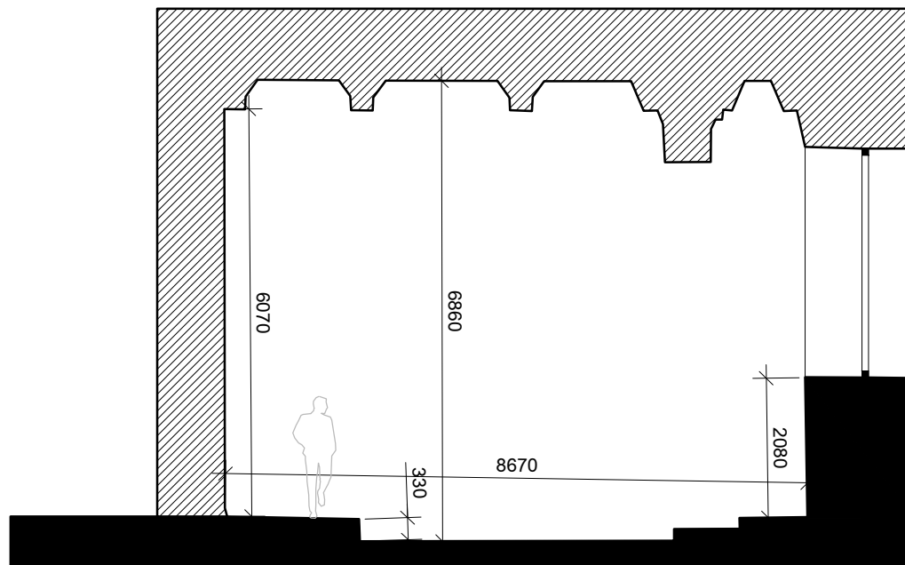
1-1
